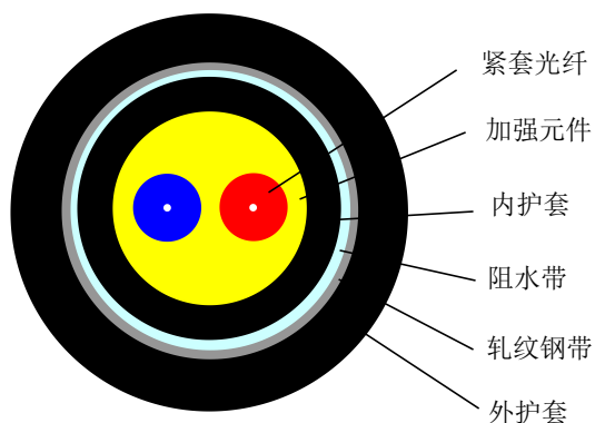
双芯圆形基站光缆 VI型
